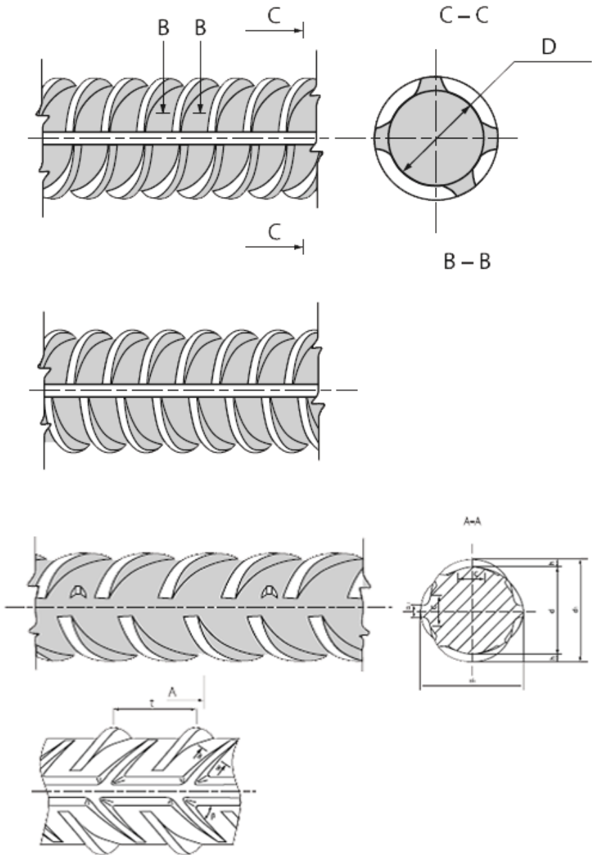
Dessin industriel de différentes structures de fer à béton
